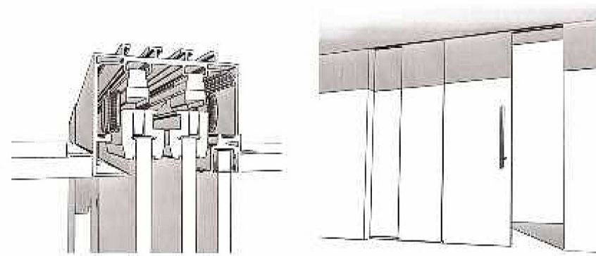
Sistema scorrevole con binario a scomparsa "SV150TM3" due o quattro ante parallele con anta fissa
