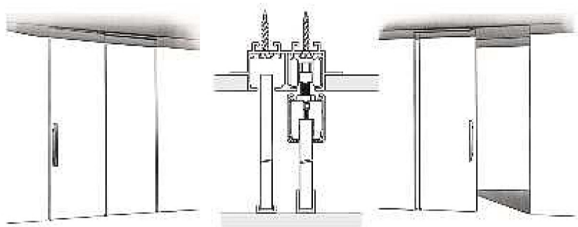
Sistema scorrevole con binario a scomparsa "TSCF 300" Due ante, una fissa e una mobile Quattro ante, due fisse e due mobili
