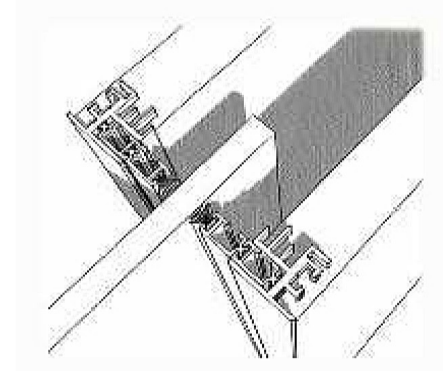
Scorrevole a scomparsa "MODULAR RASO" Telaio senza mostre da rasare adattabile a controlelai standard Anta singola Mod. Trasparente_Collezione TRASPARENTI
