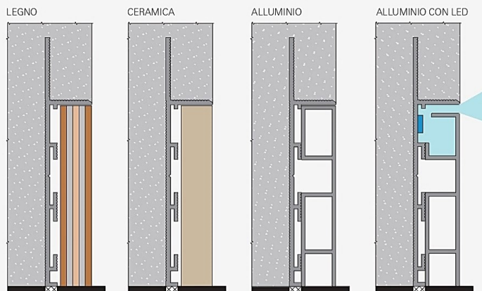
Battiscopa filo muro LED
