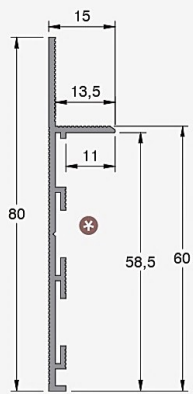
Battiscopa filo muro
